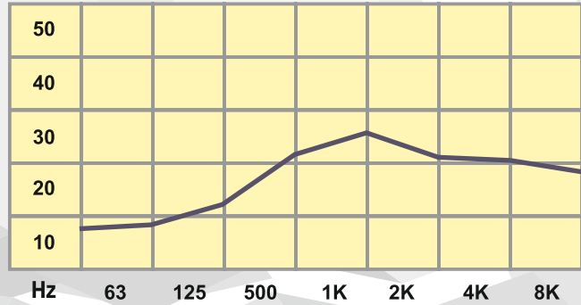
Db ATENUACIÓN ACÚSTICA (RBT 30)
