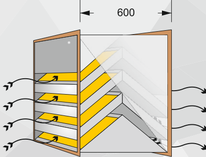
REJILLA DE 600 MM
