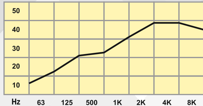
Db ATENUACION ACÚSTICA (RBT 60)
