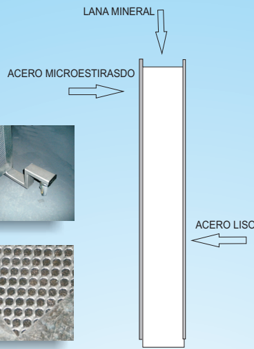
BARRERA DE PASILLO
