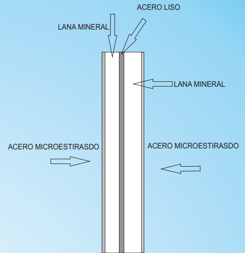
BARRERA ENTRE PUESTOS DE TRABAJO
